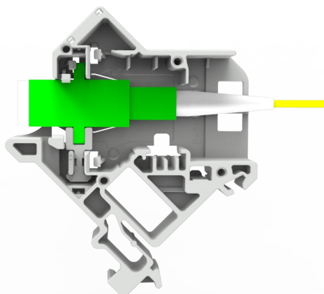
Bestückt mit CobiNet LWL Adapter LC DX
