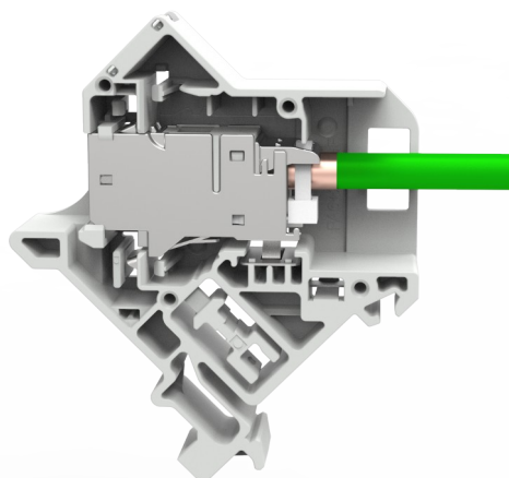
Bestückt mit CobiNet KS RJ45 Buchse
